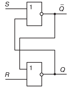
Рис. 4.11. Логическая схема RS-триггера
