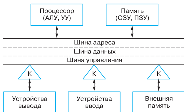
Рис. 2.7. Функциональная схема компьютера (К — контроллер)
