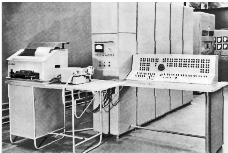
Рис. 2.6. ЭВМ «Сетунь»
